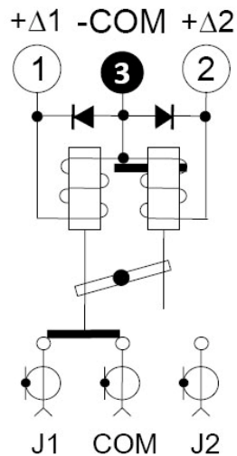
自保持（脉冲）
