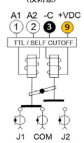
TTL和自切断 (仅闭锁)
