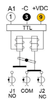
失效保护 TTL
