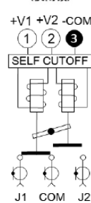
自切断 (仅闭锁)
