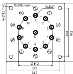
机械图纸(单位: mm) H = 50 (max) (标准) = 60 (max) (带TTL) = 65 (max) (带指示器)
